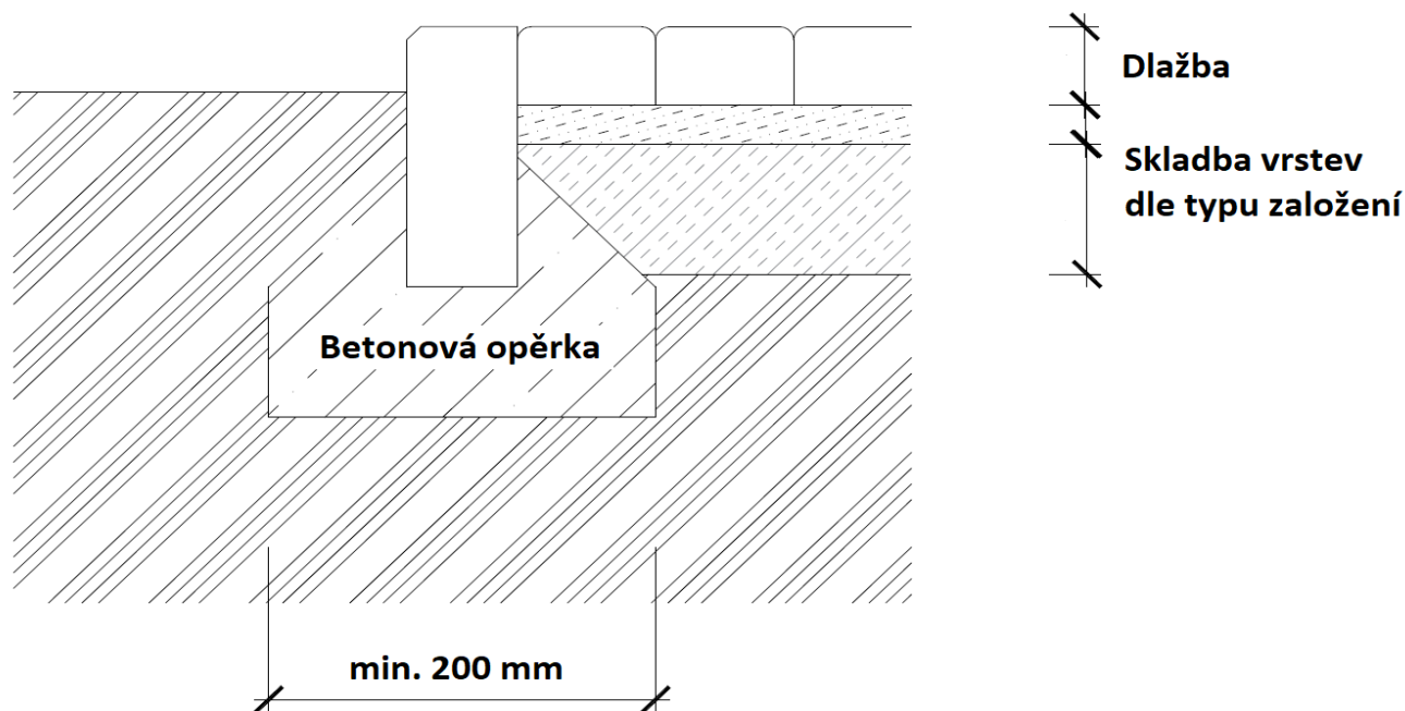
Obr. 1 – Schéma uložení parkového obrubníku
