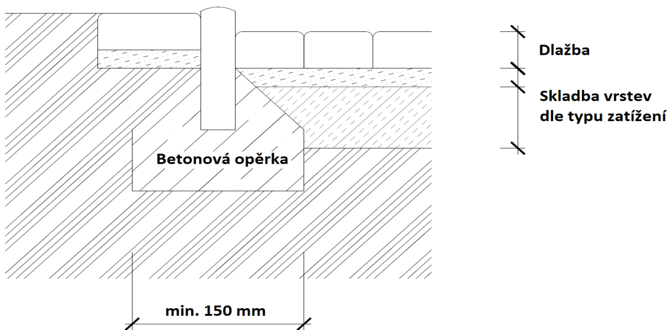
Obr. 2 – Schéma uložení zahradního obrubníku
