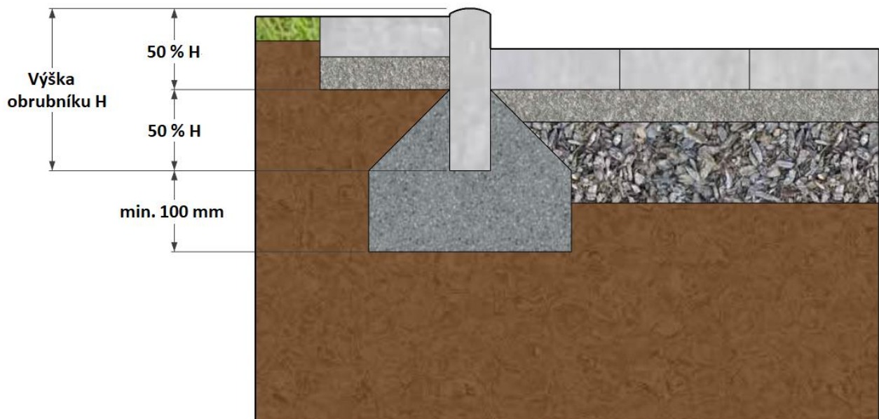
Obr. 3: Schéma osazení parkového obrubníku
