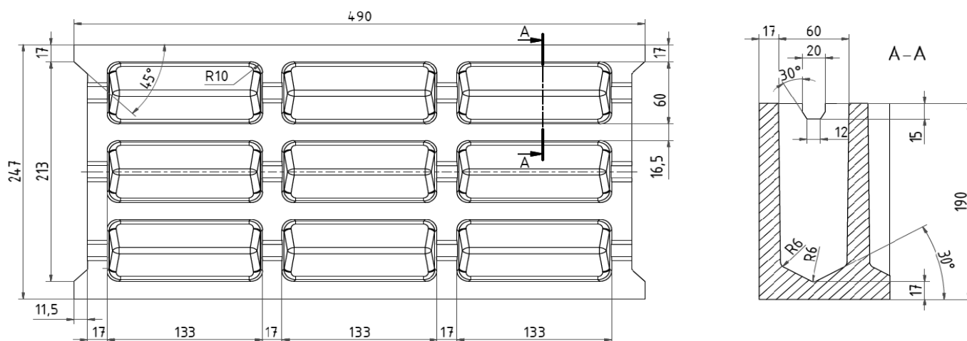
Zdící tvarovka 50/25/20 - průběžná
