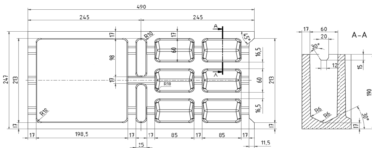
Zdící tvarovka 50/25/20 - rohová-dělicí
