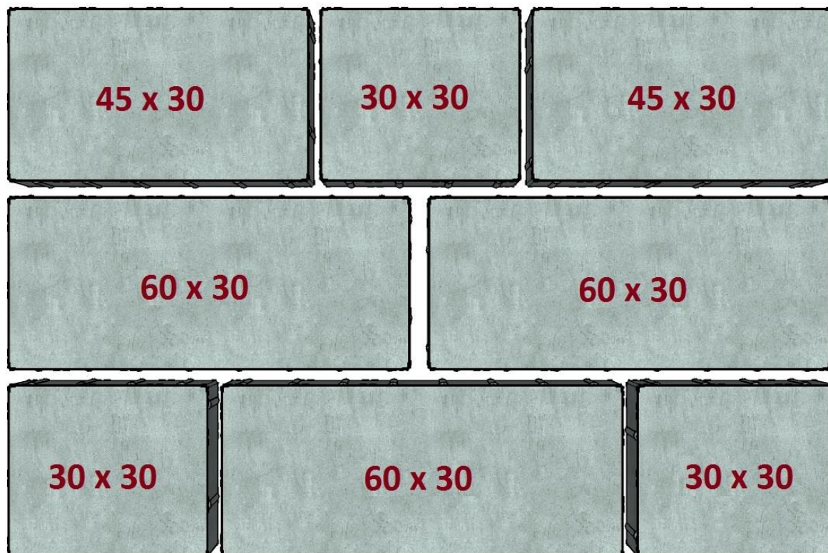
Obr. 1 - Skladba vrstvy na paletě
