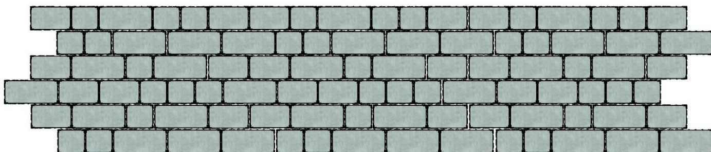
Obr. 4 – Návrh skladby položení dlažby Lazurit pro plochu širší než 2,4 m
