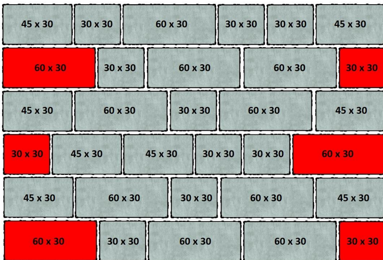
Obr. 3 – Návrh skladby položení dlažby Lazurit pro plochu širší než 2,4 m
