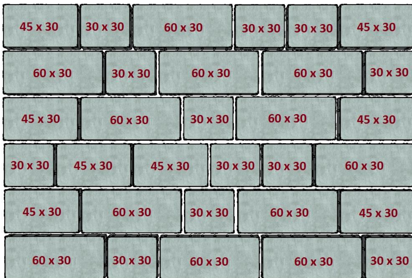
Obr. 2 – Návrh skladby položení dlažby Lazurit
