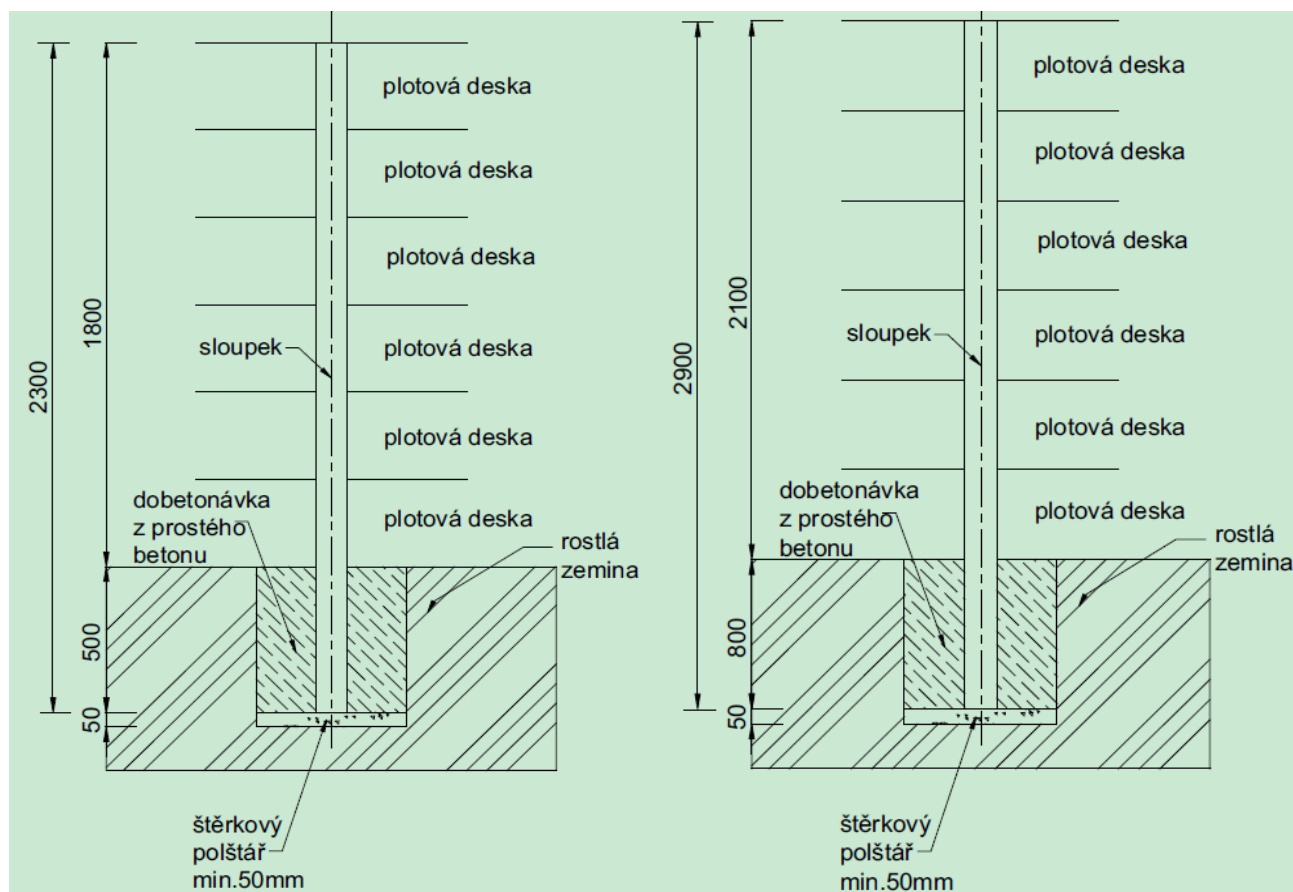
Obrázek 2 Příklad osazení sloupků v rovinném terénu
