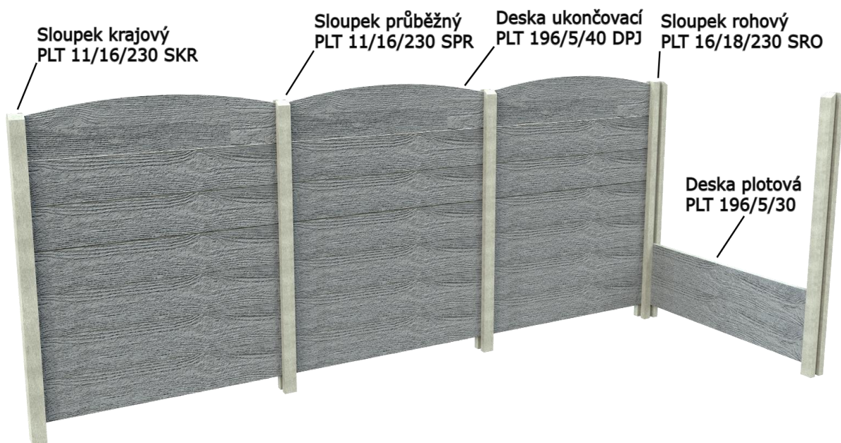
Obrázek 4 Příklad skladby plotu
