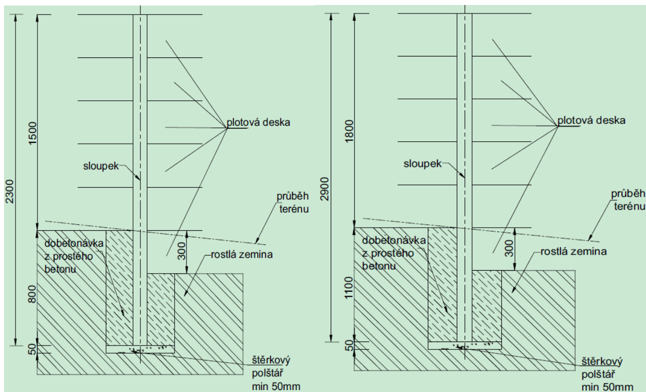
Obrázek 3 Příklad osazení sloupků ve svažitém terénu
