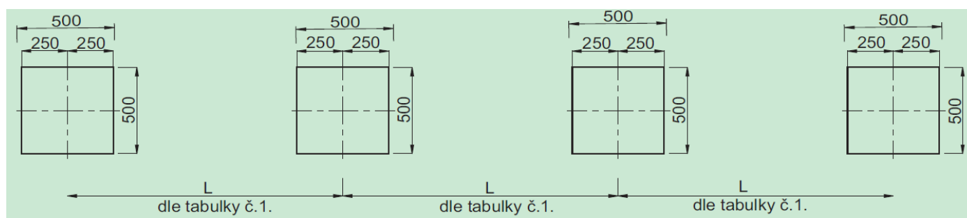
Obrázek 1 Rozmístění a tvar výkopů pro dané rozteče sloupků
