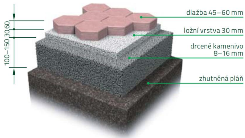
Obr. 1 – Příklad skladby chodníku
