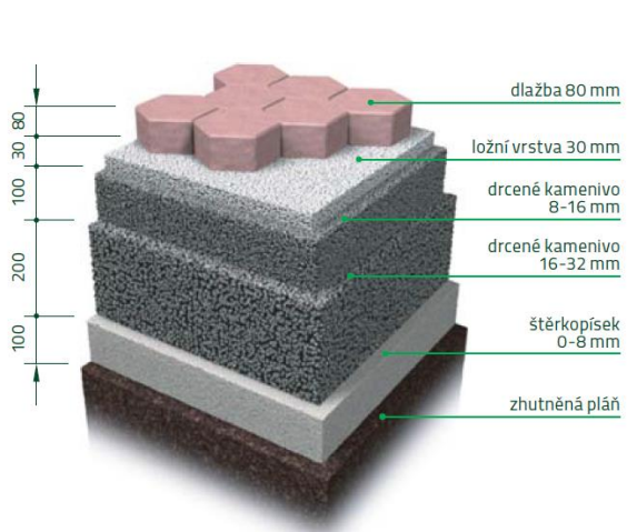
Obr. 2 – Př. skladby pojezdové plochy do 3,5 t
