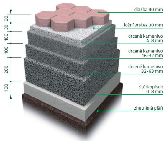
Obr. 3 – Př. skladby pojezdové plochy nad 3,5 t
