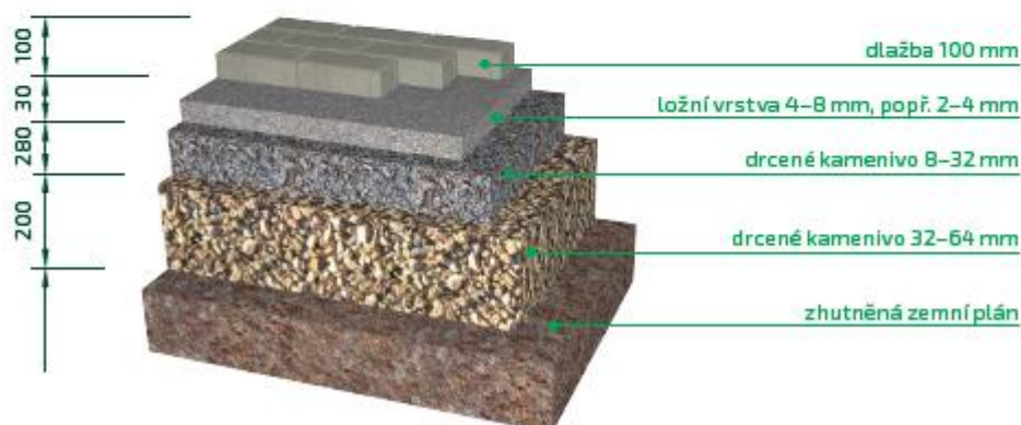
Příklad skladby pojezdové plochy pro vozidla nad 3,5 t
