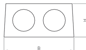
Desky vylehčené výšky 140 mm
